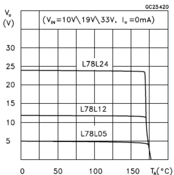
Figure3.4.6. L78L05/12/24 Thermal shutdown
