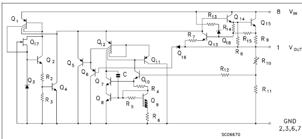
Figure3.4.1. Schematic
